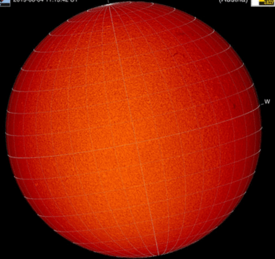
H-alpha 2019-08-04
